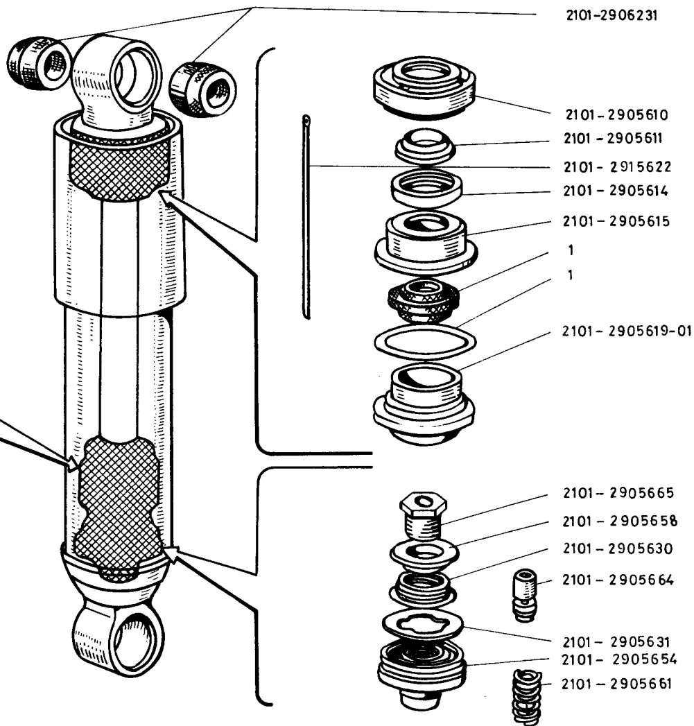
75. tábla HÁTSÓ LENGÉSCSILLAPÍTÓ - 283 -
