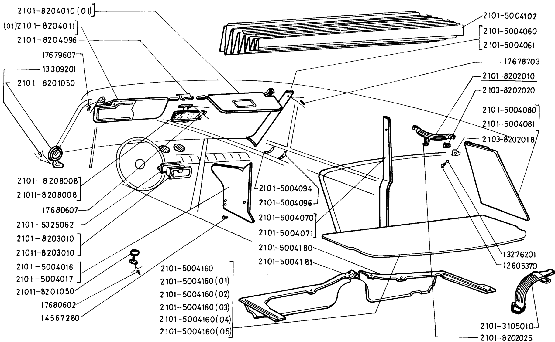
133. tábla KOCSISZEKRÉNY TARTOZÉKAI ÉS BELSŐ SZERELÉKEI
