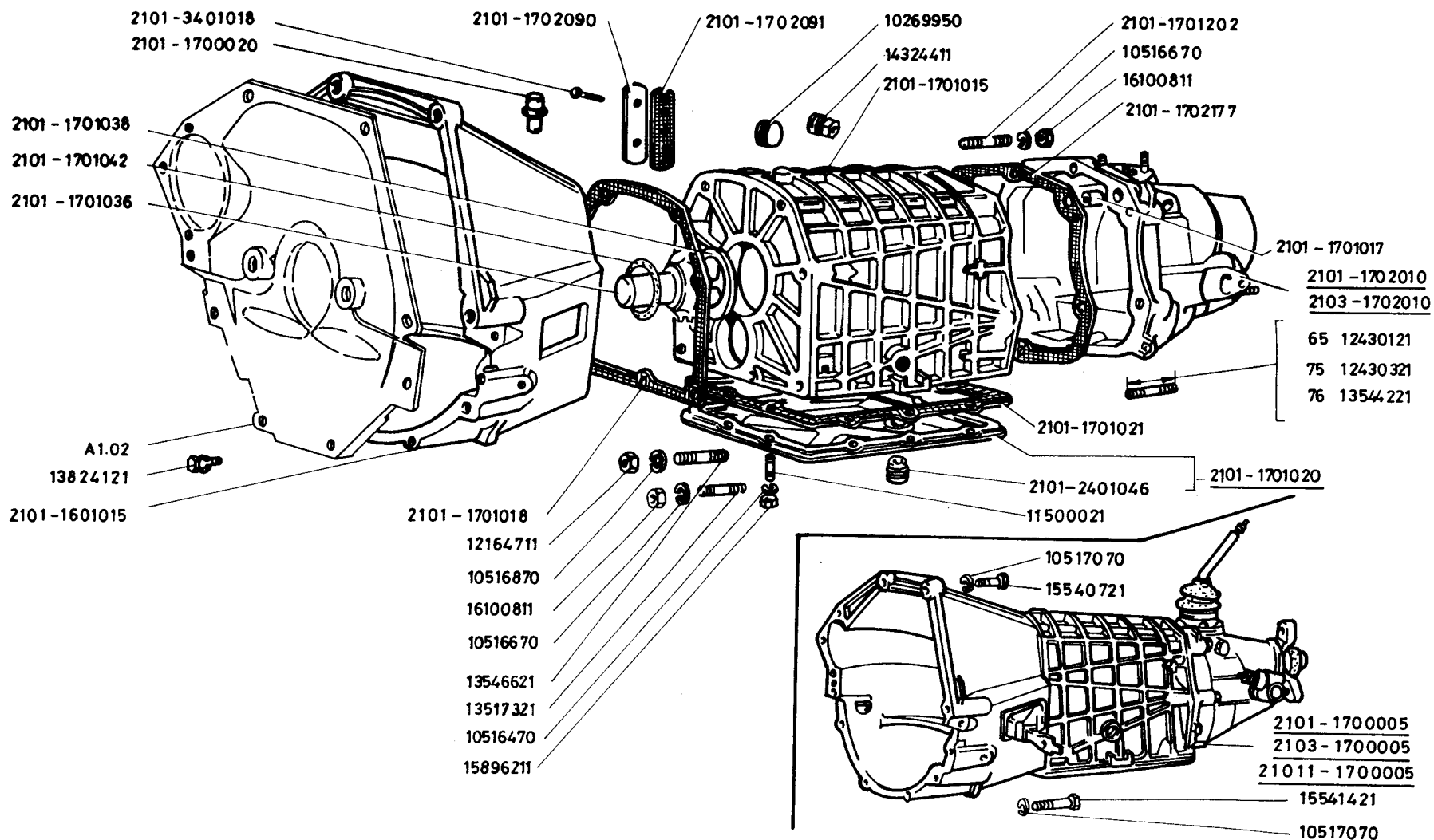
40. tábla SEBESSÉGVÁLTÓ SZEKRÉNY
